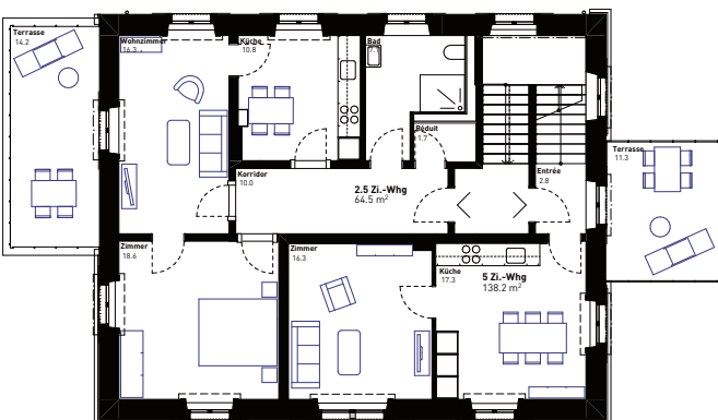
1. Obergeschoss – Villa
