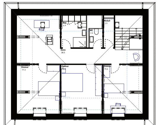
2. Obergeschoss – Villa
