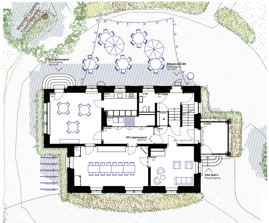
Erdgeschoss – Villa
