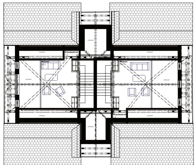
2. Obergeschoss – Riegelhaus
