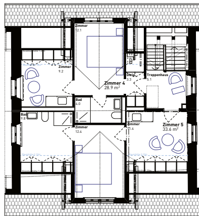
2. Obergeschoss – Kosthaus
