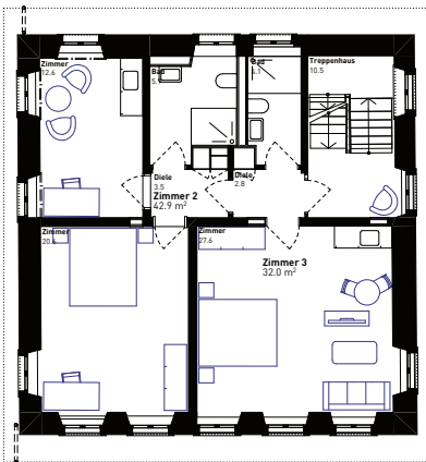
1. Obergeschoss – Kosthaus
