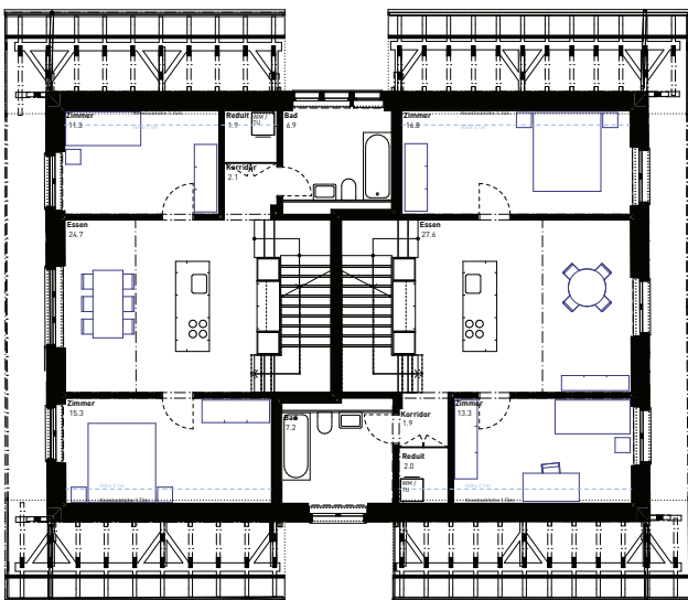
1. Obergeschoss – Riegelhaus
